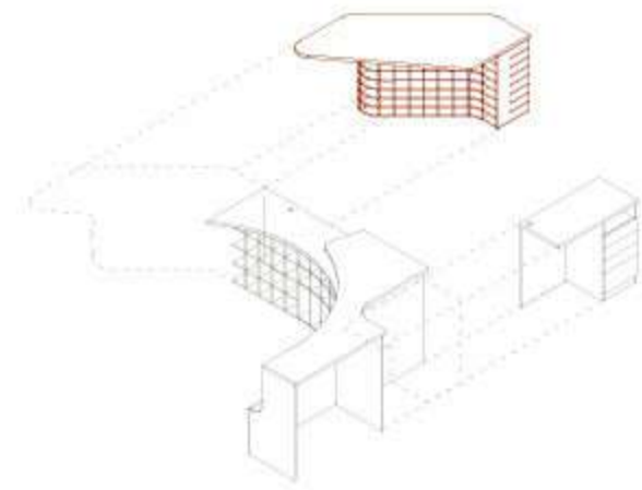
Modulo de Mostrador A
