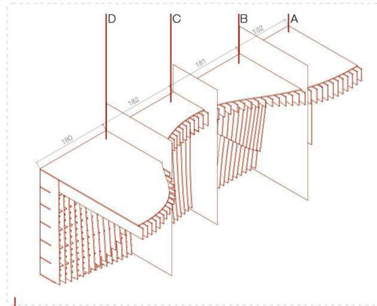
División de estantería en 4 módulos para agilizar su viabilidad y maniobración
