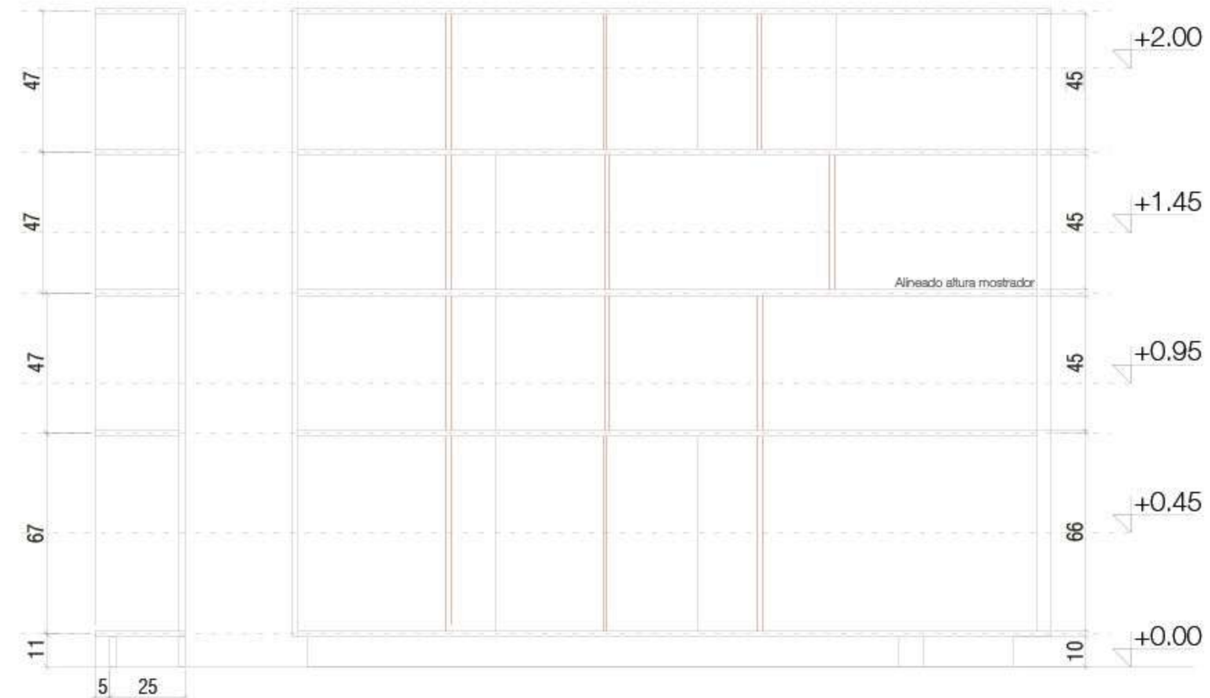
CORTE TRANSVERSAL
