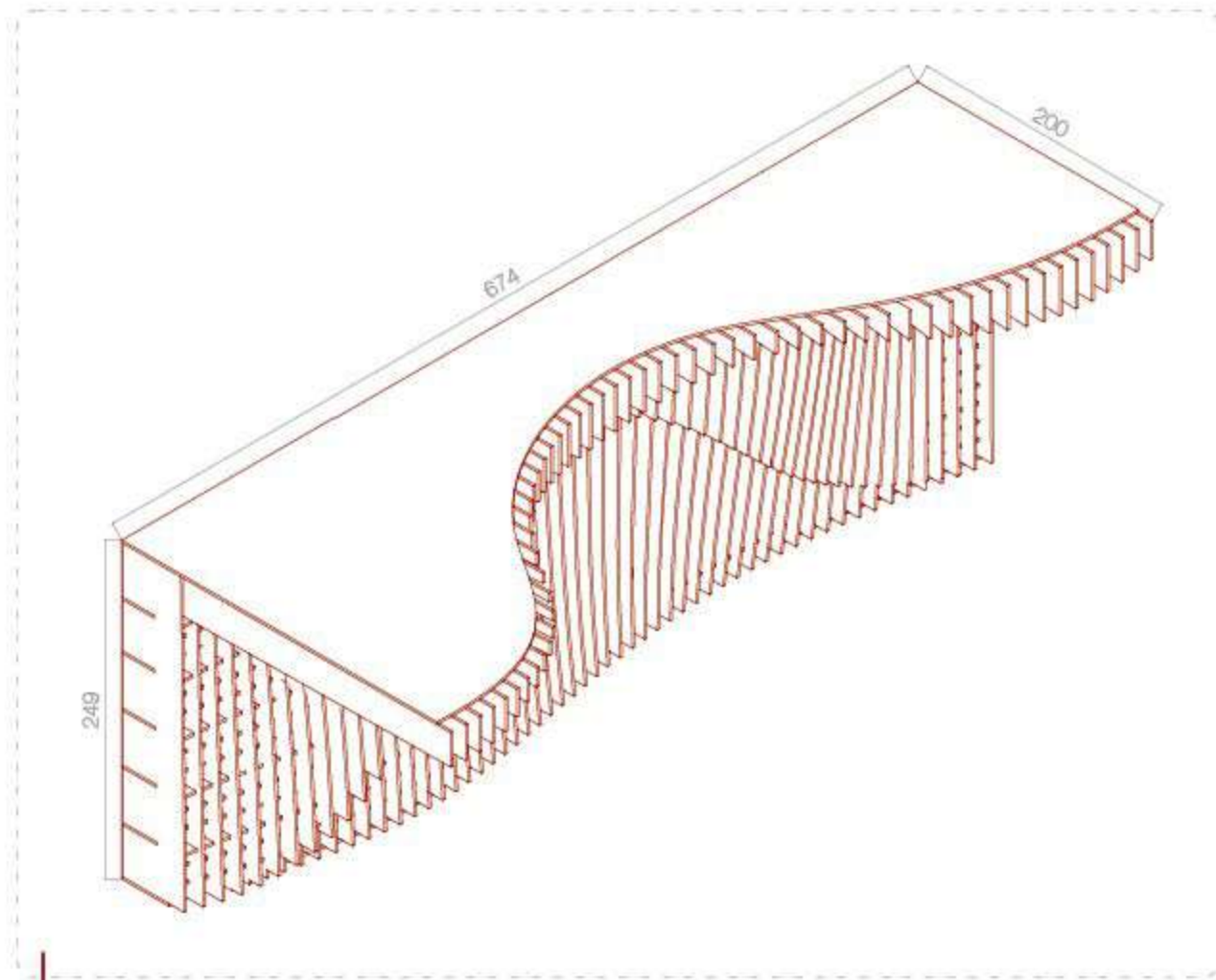
Mueble exhibidor completo
